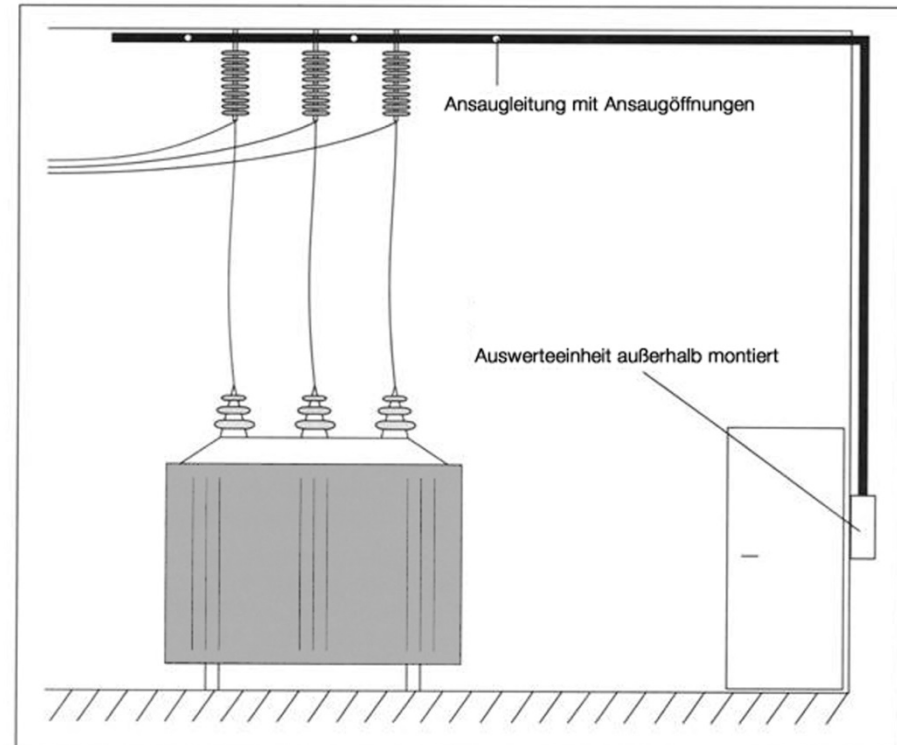
Vollständige Überwachung mit Ansaugrauchmelder
